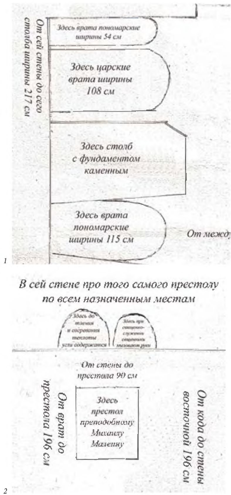
Рис. 3. Фрагменты 1, 2 чертежа алтарной зоны. ГБУТО ГА в г. Тобольске Ф. И156, Оп.1, Д.1351. Лист 13а, оригинал и перевод.
